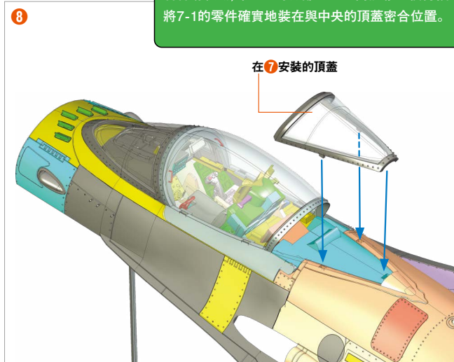
將在 7 組好的頂蓋插入在 6 組好的機身後部圖片位置。
