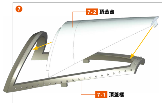
在 7-1 頂蓋框將 7-2 頂蓋窗如圖片一樣地插入。
