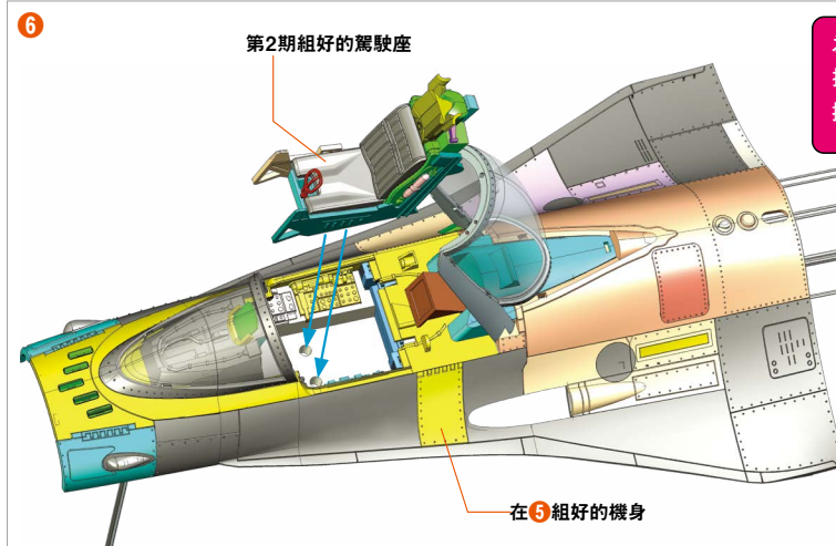
將第2期組好的駕駛座插入在 5 組好的機身圖片位置。
