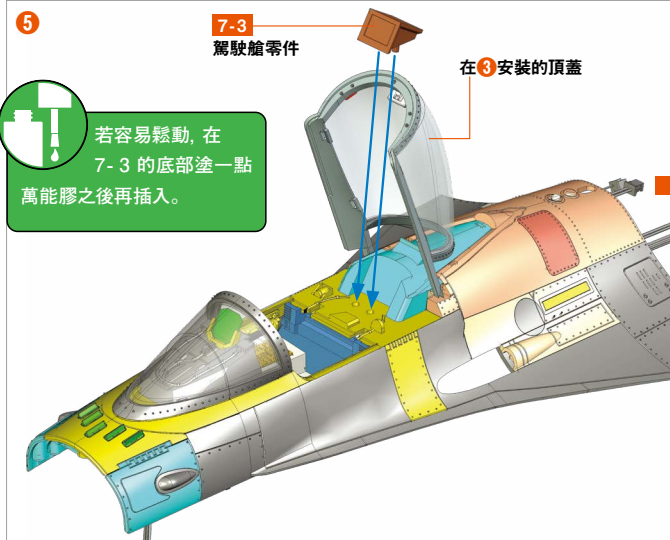
打開在 3 安裝好的頂蓋, 在圖片位置插入 7-3 駕駛艙零件。
