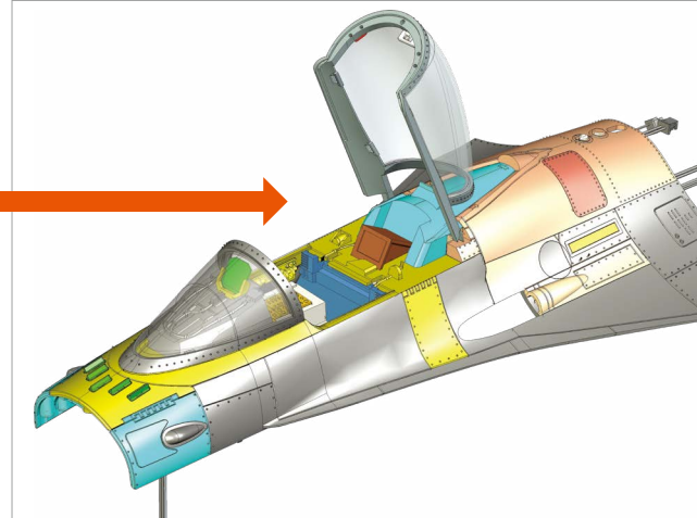
打開在 3 安裝好的頂蓋, 在圖片位置插入 7-3 駕駛艙零件。
