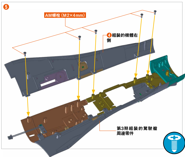
④組裝的機體右側與第3期組裝的駕駛艙周邊零件組合在一起，將圖片位置鎖上5處的AM螺栓 (M 2.0×4 mm)
